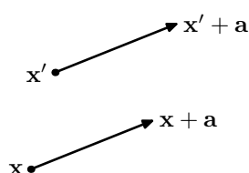
図 2.1 平行移動
