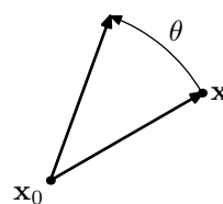
図 2.2 回転
