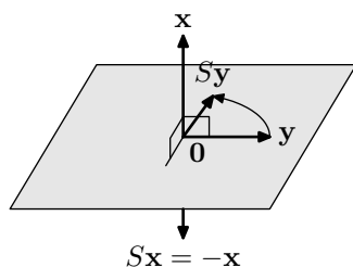
図 1.23 鏡映と回転
