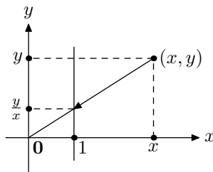
図 3.23 透視投影
