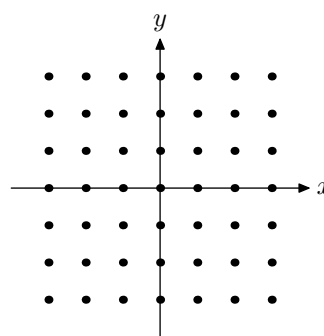
図 2.8 \mathbf{Z}^n
