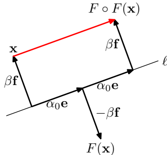
図 2.90 並進鏡映
