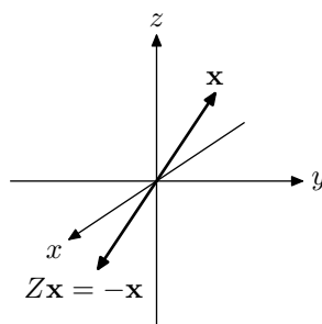
図 1.24 Z
