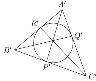
図 3.22 内接円
