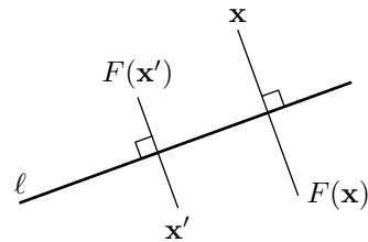
図 2.87 鏡映
