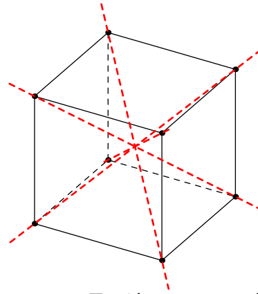
図 1.15 最も遠い二つの頂点を通る直線に沿っての 2\pi/3 回転の極
