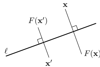
図 2.42 鏡映
