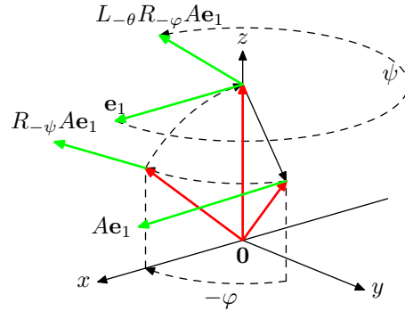
図 3.55 Euler 角: \mathbf{e}_1 の動き
