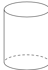
図 2.89 \mathbb{R}^3 の円柱
