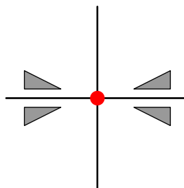
图 2.83 D_2, 0, D_2 , 万華鏡
