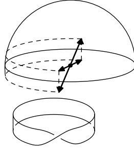
図 3.30 \mathbf{P}^2 とメビウスの帯
