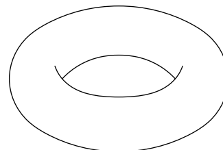
図 2.97 \mathbb{R}^3 のトーラス
