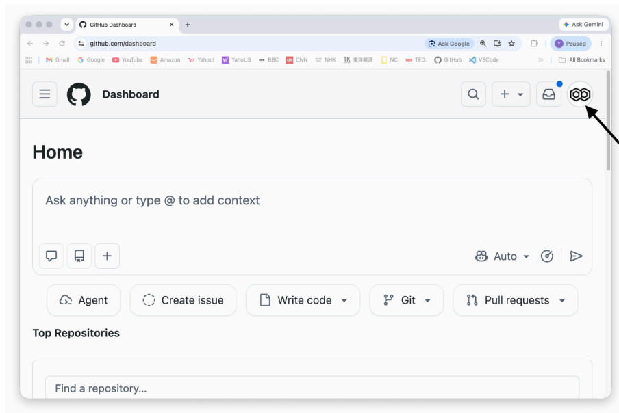
図 4. GitHub の Home
