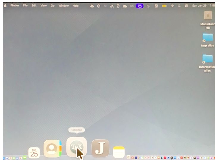
図 4. Dock の表示
