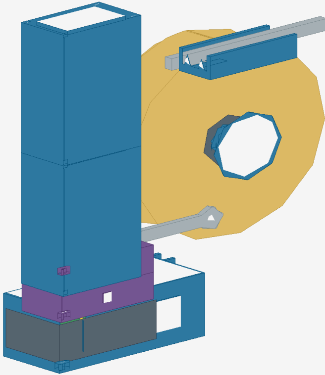
그림 7: Puller 이후 solid guide, dancer sweep, traverse와 full spool
