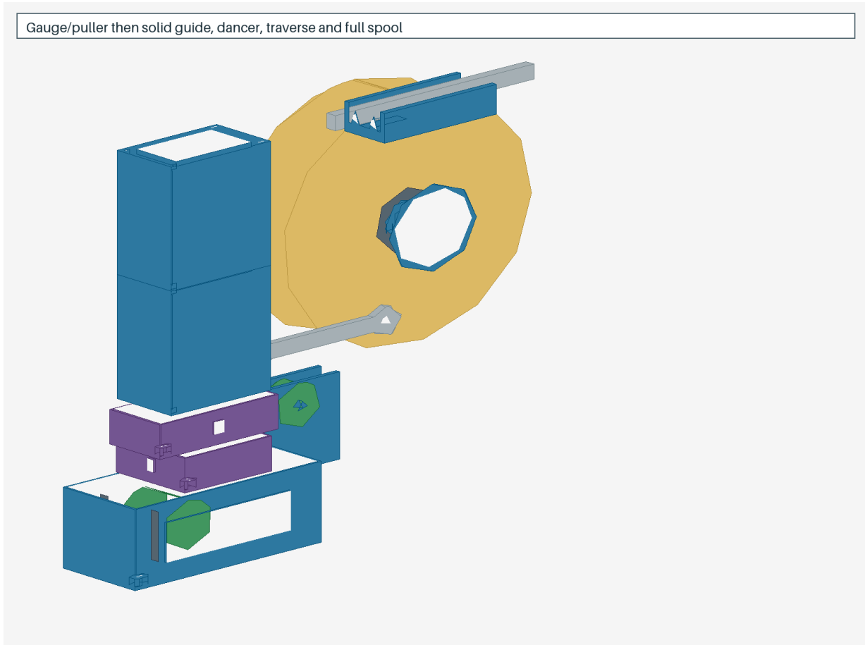
그림 6: Solid guide와 full motion spooler
