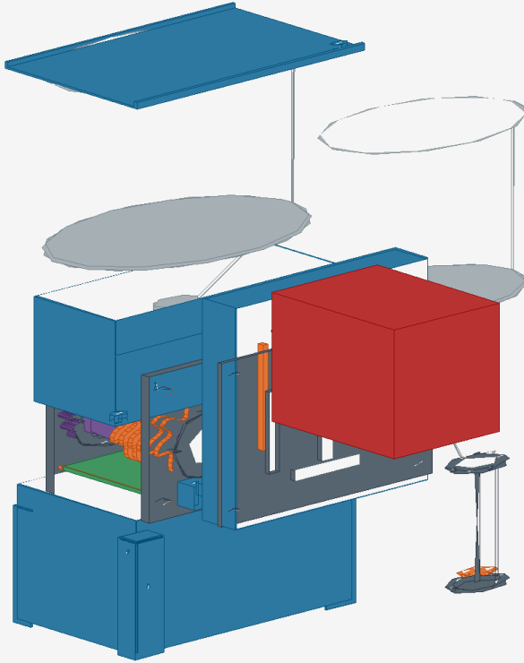
그림 5: 공용 input/cutter/screen/bin — metal shaft/bearing plate load path
