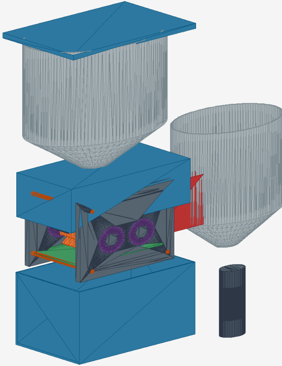
그림 3: 공용 input/cutter/screen/bin — metal shaft/bearing plate load path
