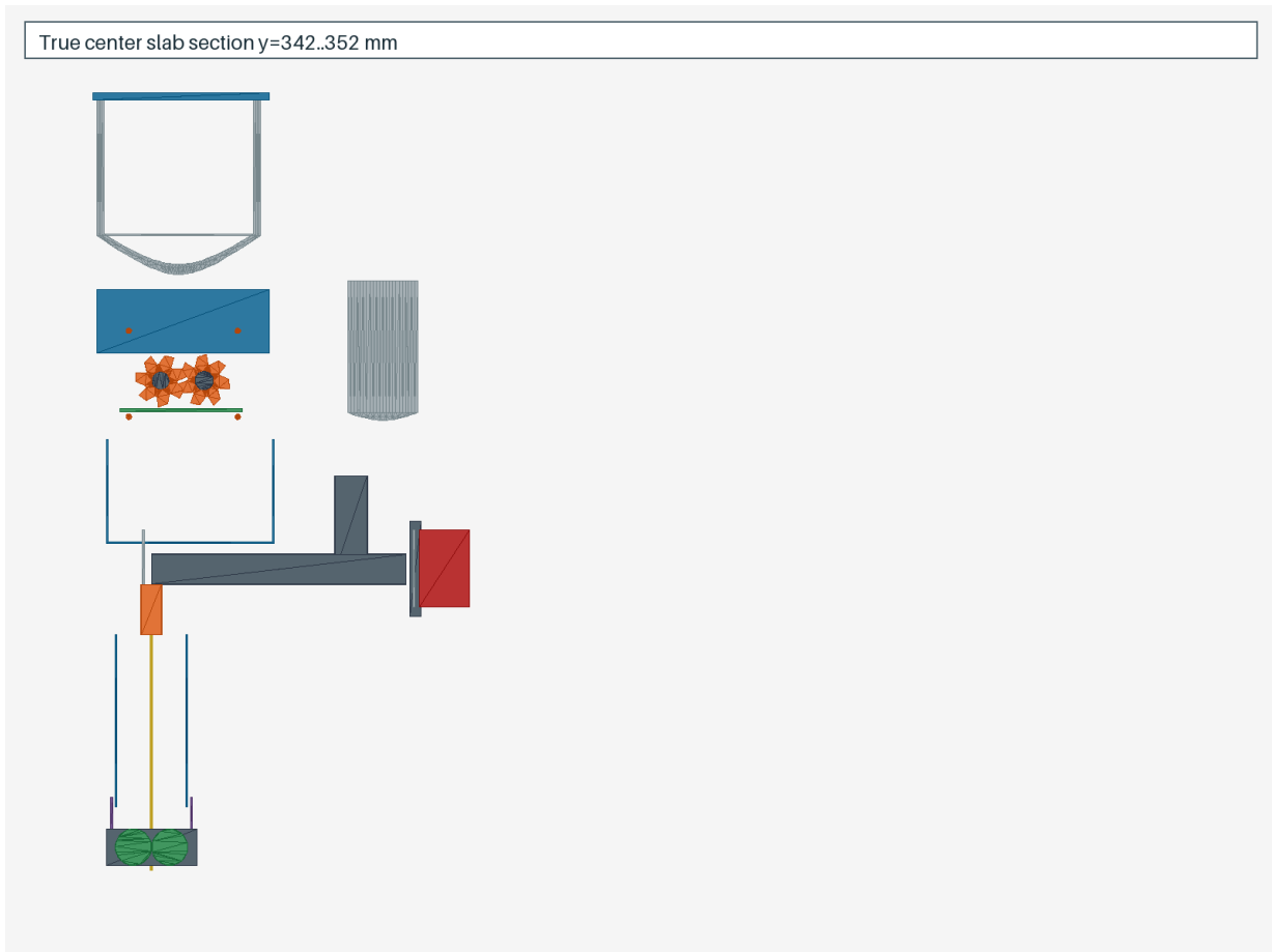
그림 4: Section — hopper/cutter와 horizontal hot zone, vertical forming
