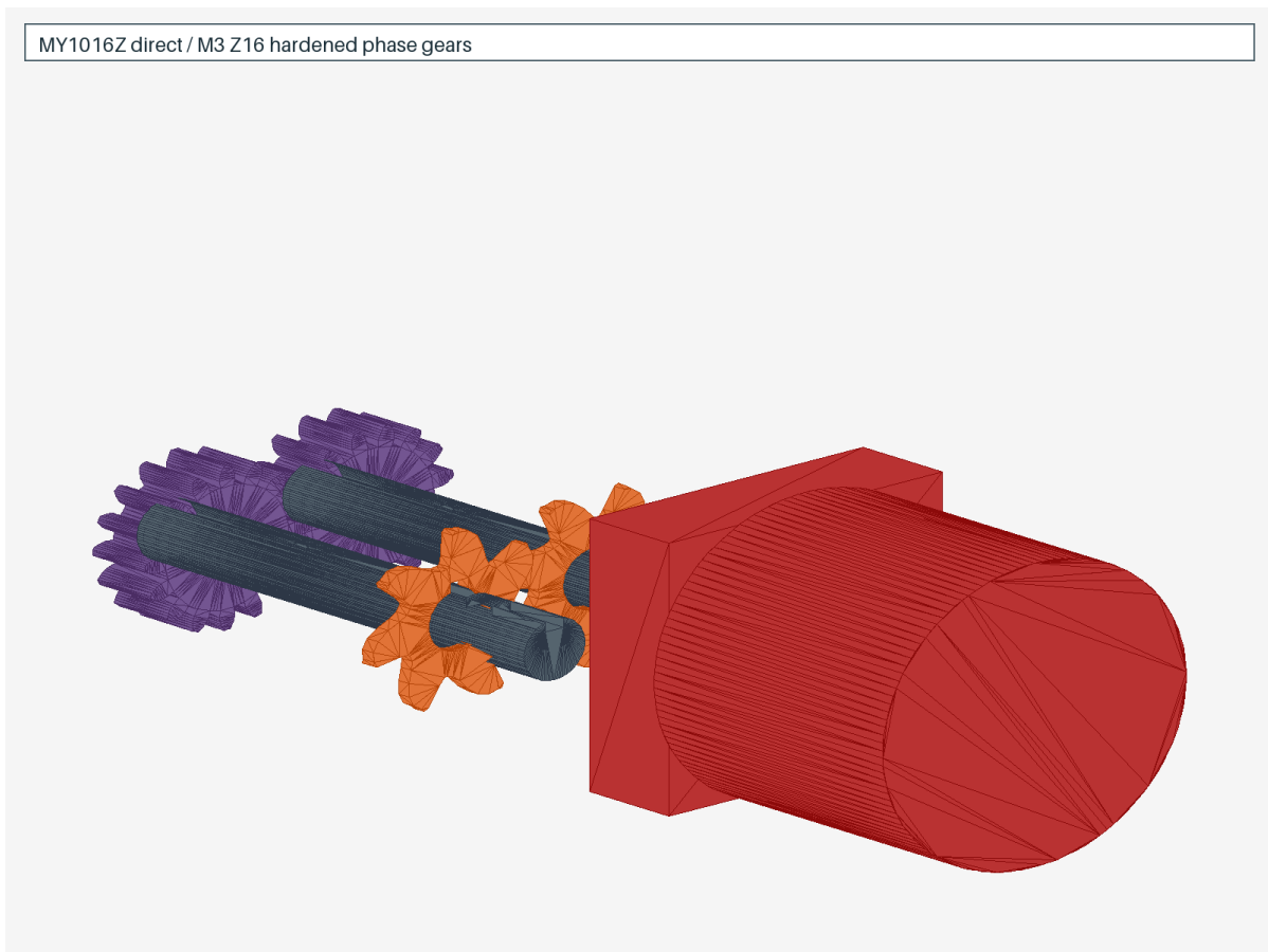
그림 4: Guard 제거 render — direct motor, ROTEX19 coupling과 hardened phase gear pair
