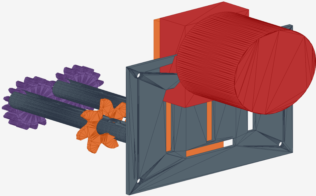
그림 3: Interchangeable donor geared-DC / 35 chain / cycloidal-derived cutter 조립 — 정상 운전은 guard 장착
