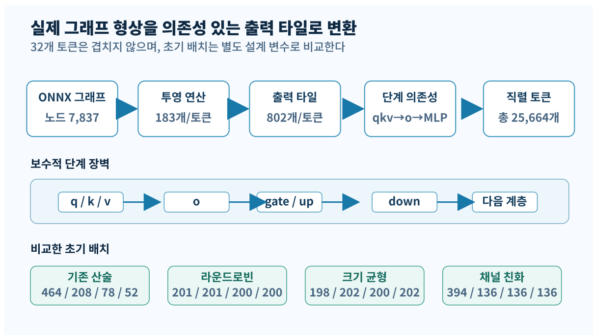
그림 2. 실제 Gemma 그래프의 투영 연산을 의존성이 있는 출력 TileJob으로 변환하는 과정. 배치 규칙은 그래프 사실이 아니라 별도 모델 변수다.
