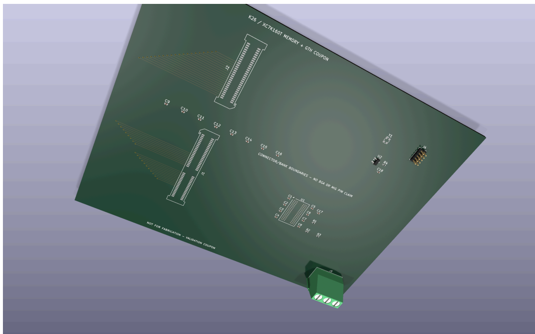
그림 7. 실제 KiCad 원본에서 렌더링한 인터페이스 라우팅 쿠폰. 두 범용 경계 커넥터, 대표 DDR3L x16 슬라이스, GTH-refclk 배선을 표시한다. NOT FOR FABRICATION.
