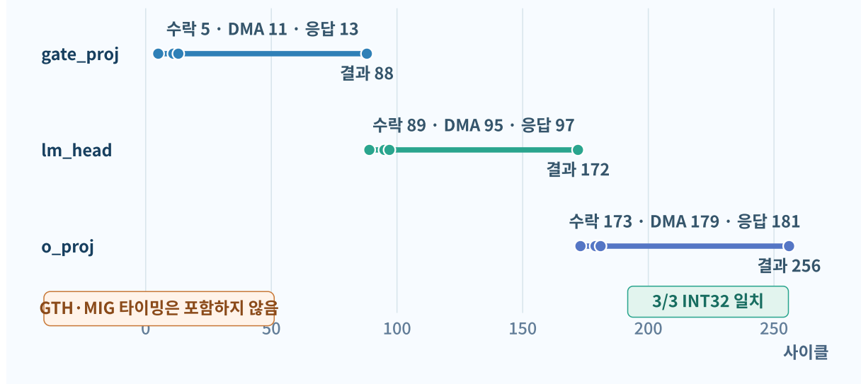
그림 4. 실제 Gemma 대표 타일 세 개가 페루프 논리 RTL 경로를 통과한 사이클 추적. 세 결과는 소프트웨어 INT32 기준과 일치한다.
