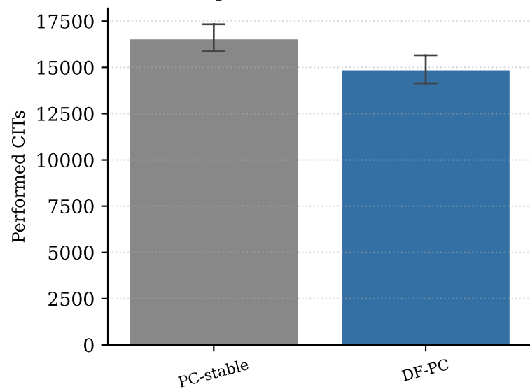
Graph=SF, Data=Linear Sem
