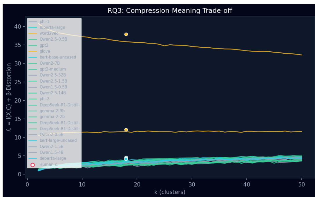
图 2: RQ3: 全部 24 个模型的叠加 \mathcal{L} 曲线。经典嵌入在独立坐标上显示。每条曲线的终点并非收敛——只是展示到 k = 50 。
