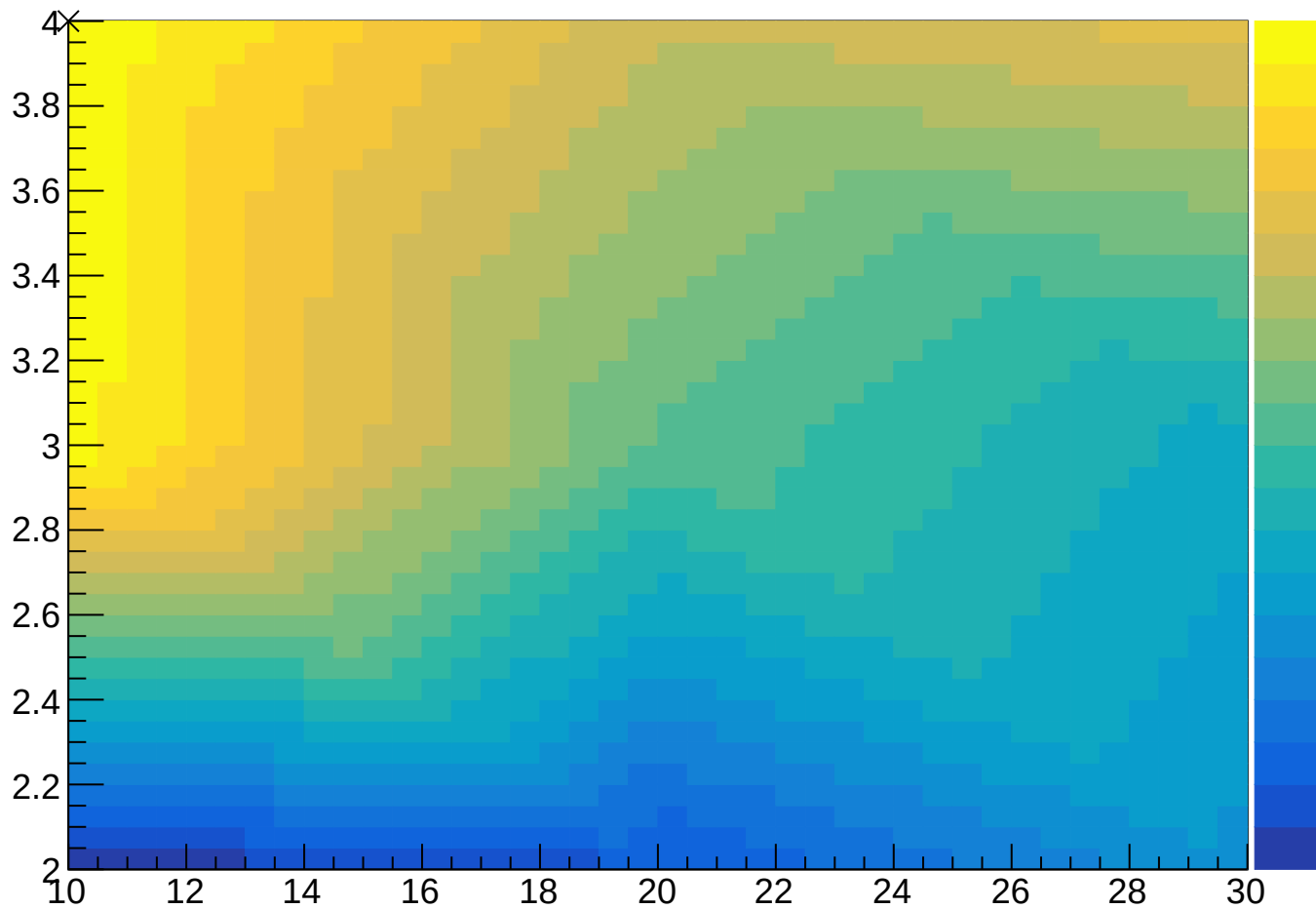
nCuts:MaxDepth
