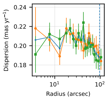
NGC 5904
