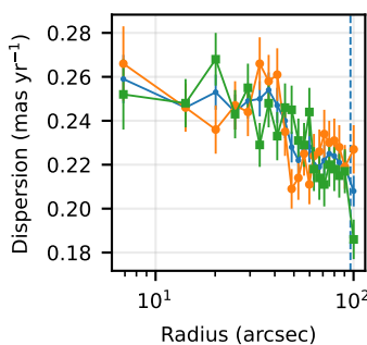
NGC 6541
