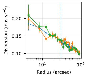
NGC 5986
