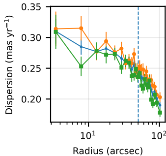
NGC 2808
