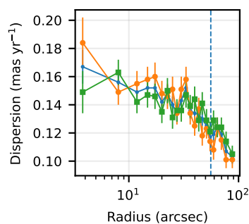
NGC 7078
