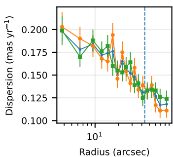
NGC 6723
