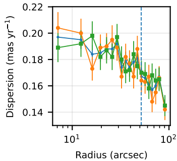
NGC 5904
