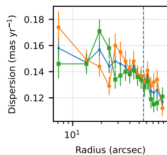
NGC 5986
