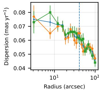
NGC 5927
