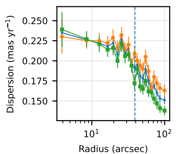
NGC 7078
