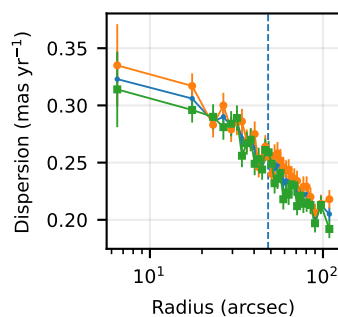
NGC 6637
