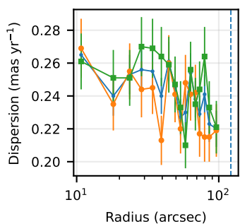
NGC 6624
