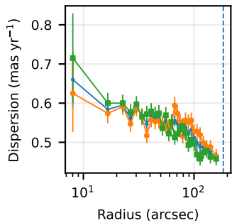
NGC 2808
