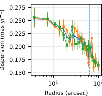
NGC 6715
