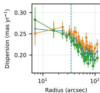
NGC 6681
