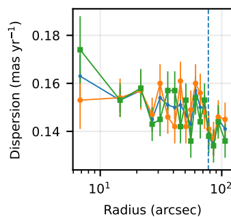
NGC 5927
