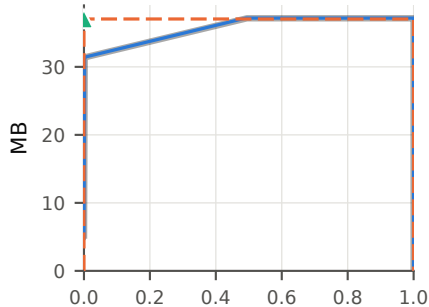
Lua
