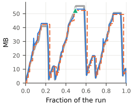
Lua
