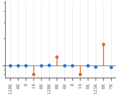
tc (scale 10)
