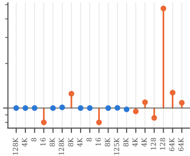
bfs (scale 10)
