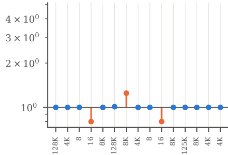
pr (scale 10)
