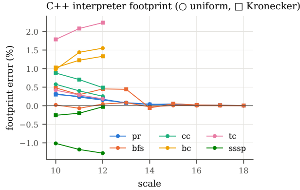
Figure 24: Footprint error of the C++ interpreter per scale.
