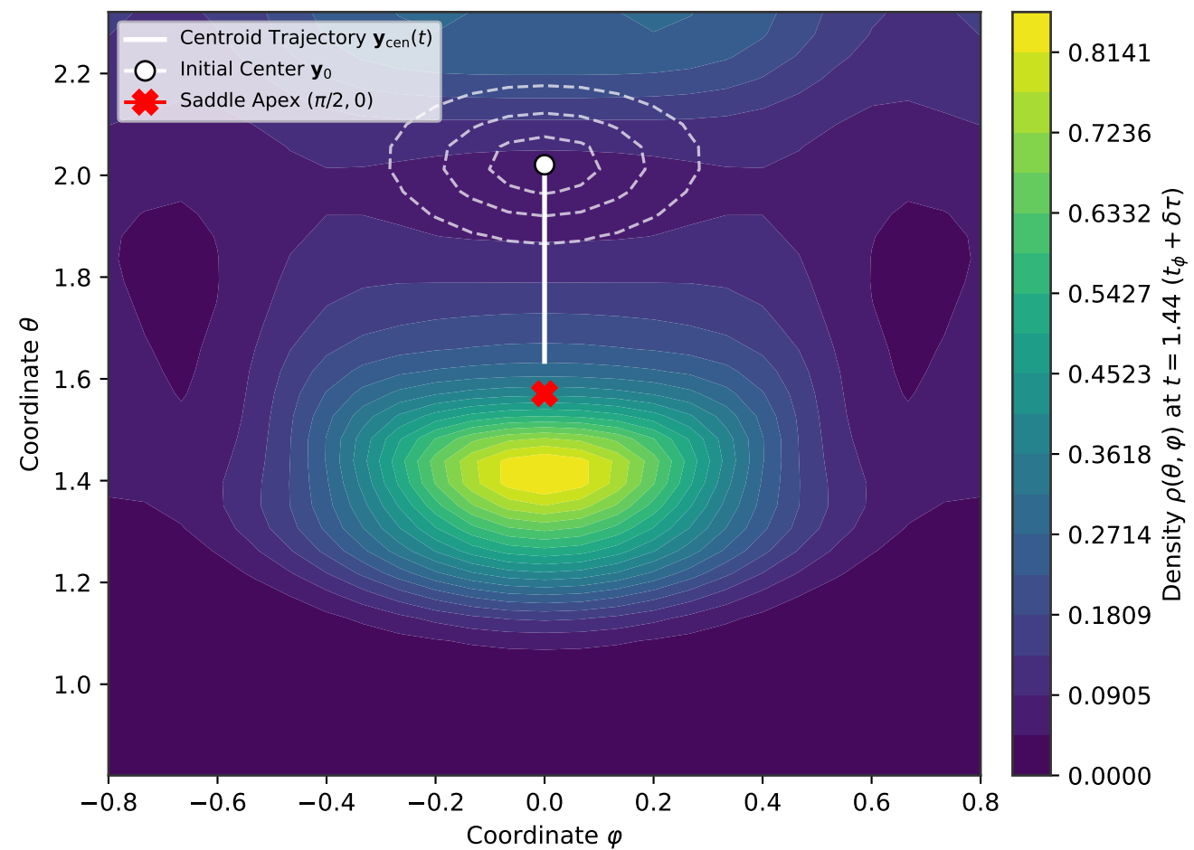
(d) Coherent Saddle Penetration Centroid Traaversal & Soliton Localization ( t = 1.44 )
