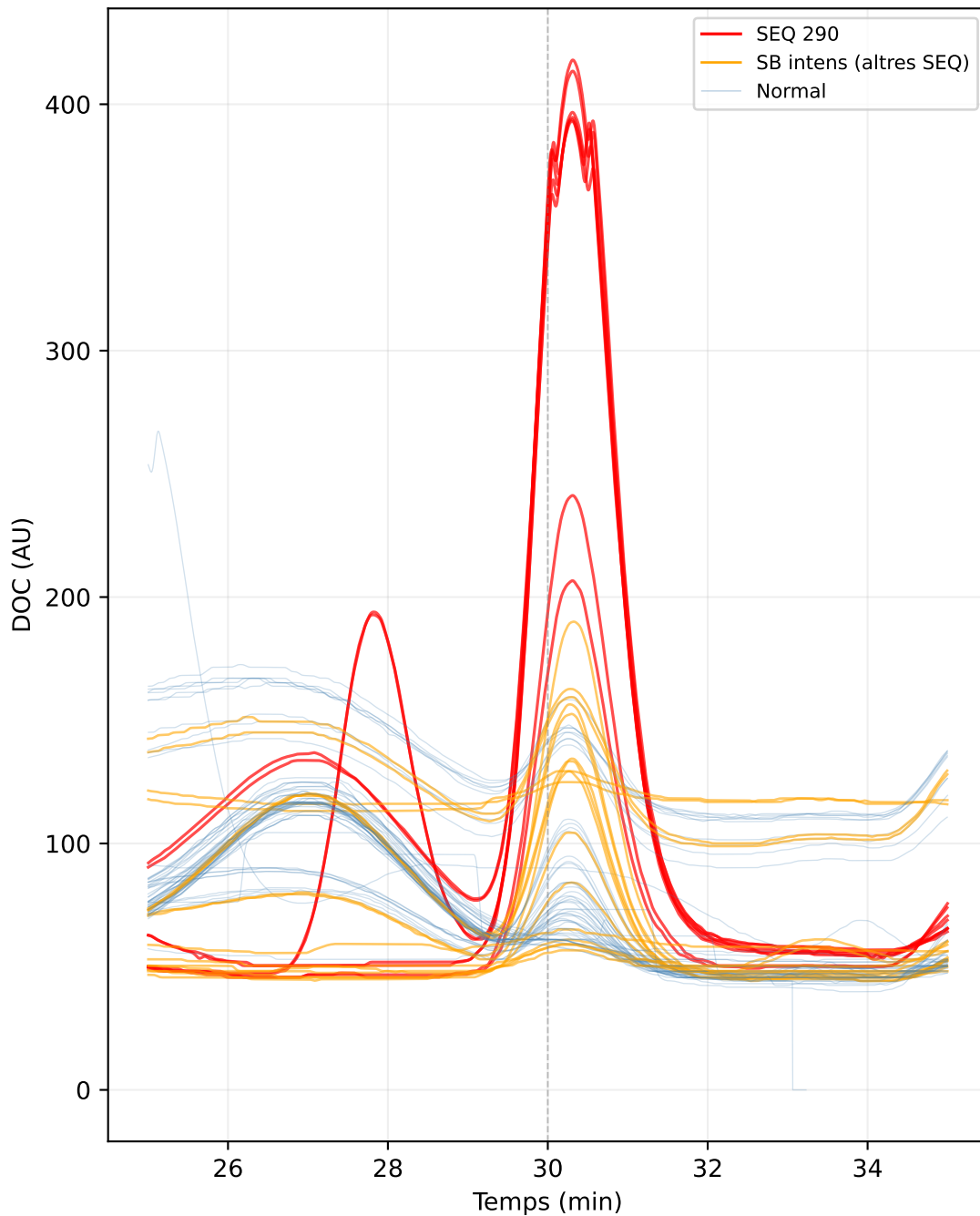
Senyal DOC (UIB)
