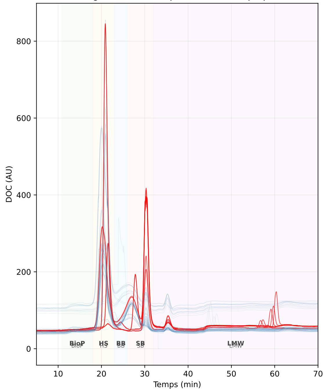
Cromatograma DOC complet — fraccions proposades
