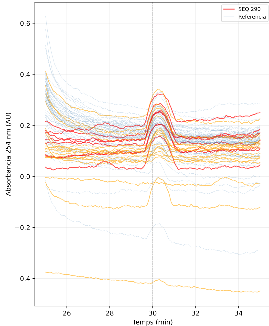
Senyal DAD 254 nm
