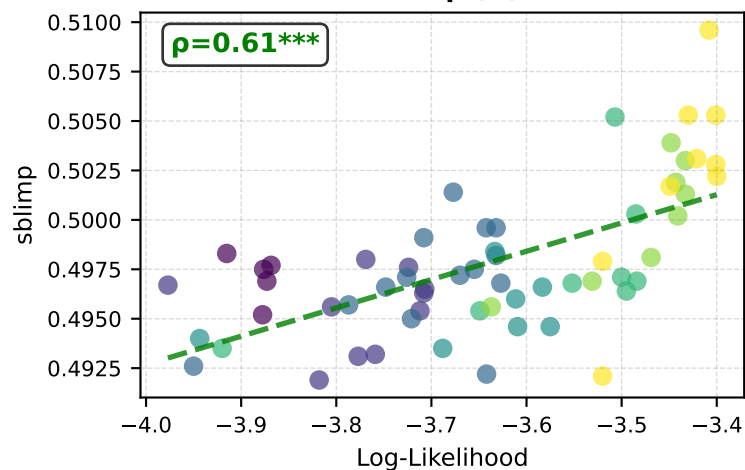
sblimp (↑)
