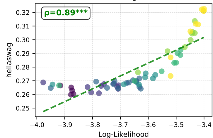
hellaswag (↑)
