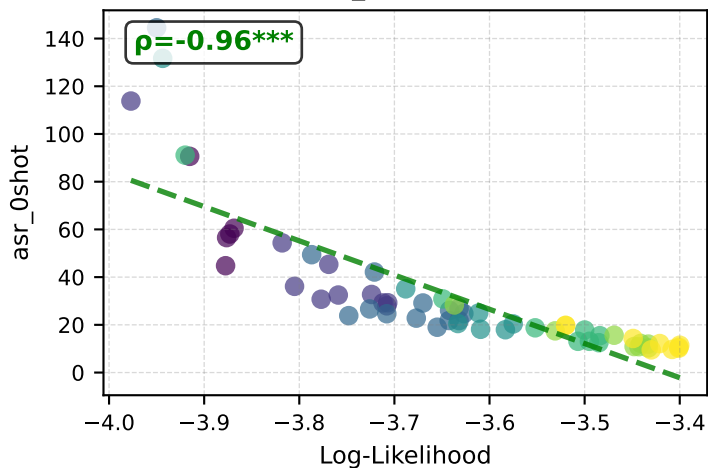
sblimp (↑)
