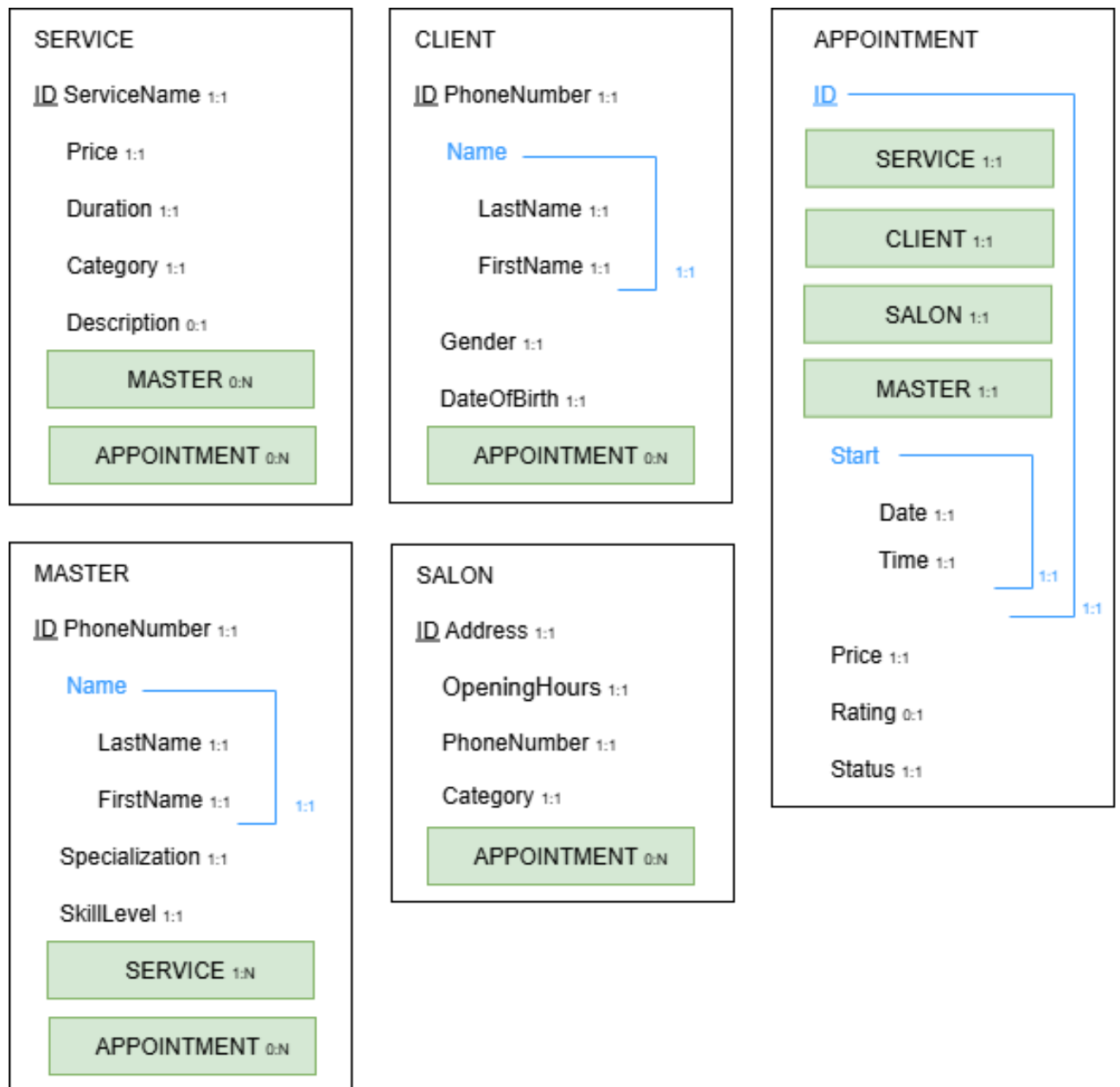
Рис. 1 — Модель семантических объектов для системы записи в салоны красоты
