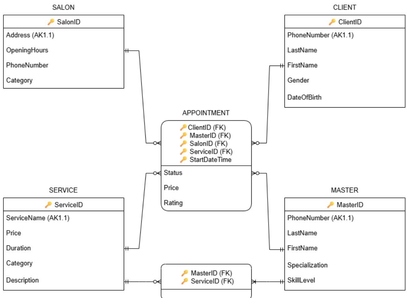
Рис. 2 — Реляционная модель для системы записи в салоны красоты, построенная по модели семантических объектов
