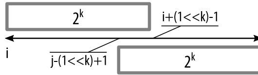
Figura 9.13: Explicación de \text{RMQ}(i, j)
