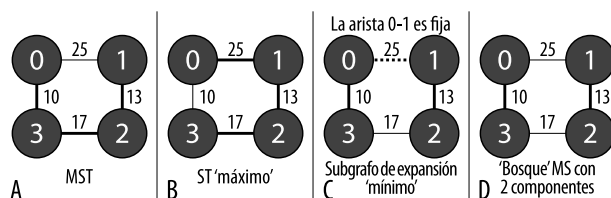
Figura 4.13: De izquierda a derecha: MST, ST 'máximo', SS 'mínimo', 'bosque' MS
