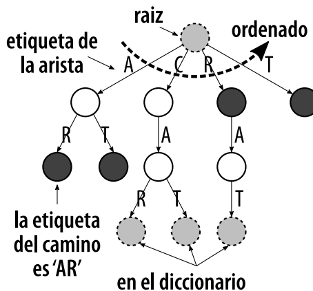
Figura 6.2: Trie de sufijos
