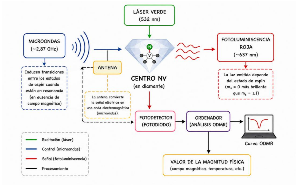
Figura 12. Montaje experimental simplificado para la técnica de ODMR basada en centros NV en diamante. Elaboración propia.
