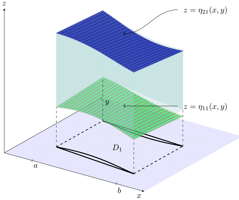
Figura 8.3: Conjunto elemental de Tipo I.
