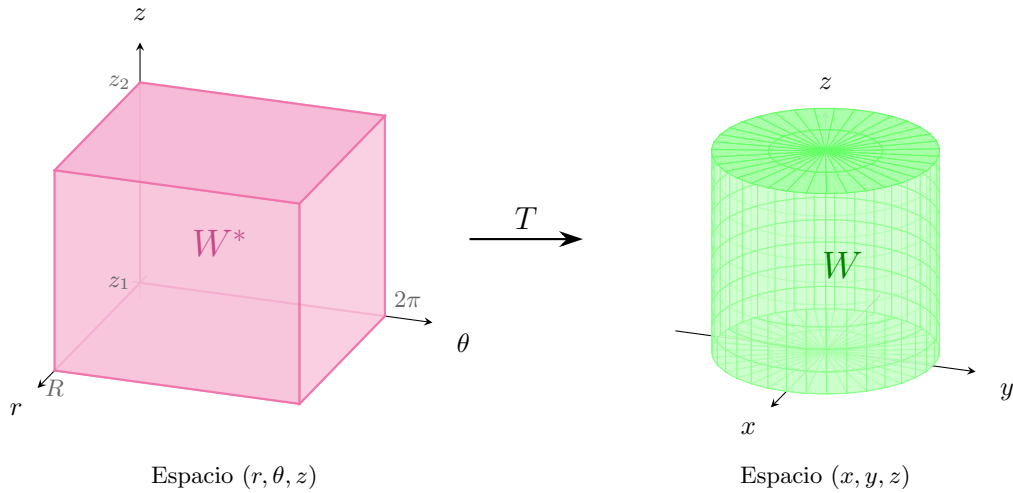
Figura 8.8: Visualización del sistema de coordenadas cilíndricas. El bloque W^* a la izquierda representa la región en el espacio (r, \theta, z) con sus límites típicos, mientras que el cilindro W a la derecha muestra cómo se transforma esa región en el espacio (x, y, z) mediante la transformación T . Ver en GeoGebra
