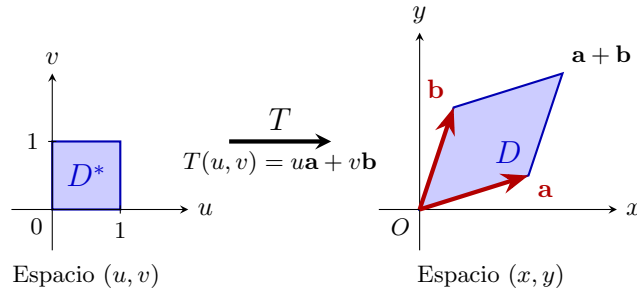
Figura 8.2: Puede observarse que el cuadrado D^* en el espacio (u, v) se transforma en un paralelogramo D en el espacio (x, y) bajo la transformación lineal T .
