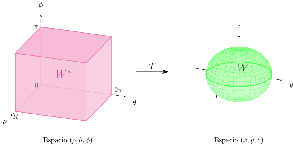
Figura 8.7: Visualización del sistema de coordenadas esféricas. El bloque W^* a la izquierda representa la región en el espacio (\rho, \theta, \phi) con sus límites típicos, mientras que la esfera W a la derecha muestra cómo se transforma esa región en el espacio (x, y, z) mediante la transformación T . Ver en GeoGebra
