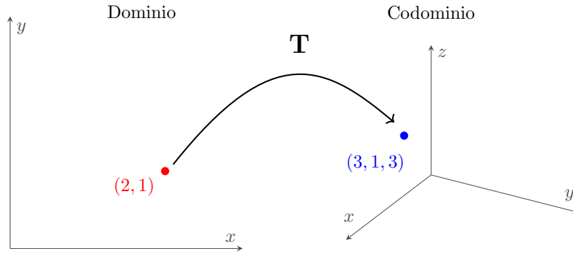
Figura 1.14: Visualización de (2, 1) y \mathbf{T}(2, 1) = (3, 1, 3) .
