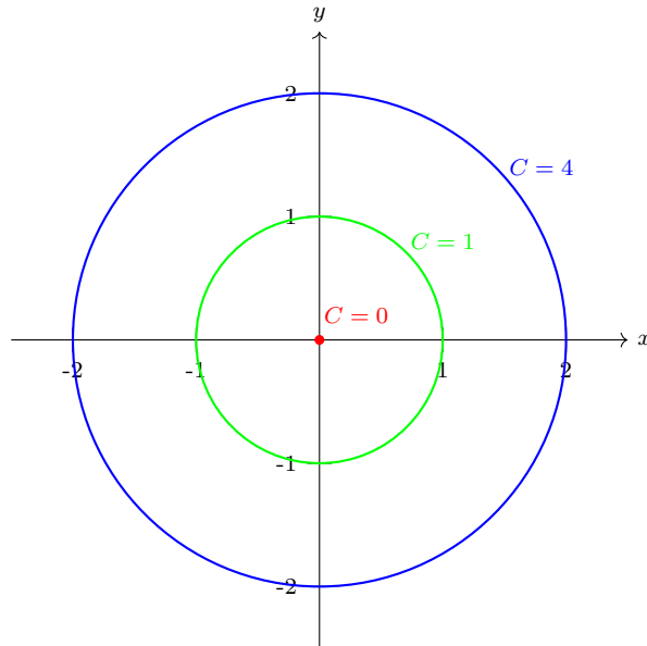
Figura 1.17: En rojo, verde y azul los conjuntos C(0, f) , C(1, f) y C(4, f) , respectivamente.
