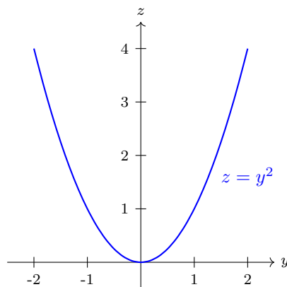
Figura 1.19: En azul la relación z = y^2 y x = 0 .
