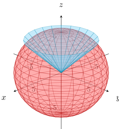
Figura 1.26: Representación de la región pedida. Ver en GeoGebra
