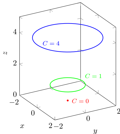
Figura 1.18: En rojo, verde y azul los cortes de \text{Graf}(f) con los planos horizontales z = 0 , z = 1 y z = 4 , respectivamente.
