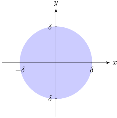
Bola con distancia inducida por la norma 2 Bola con distancia inducida por la norma 1
