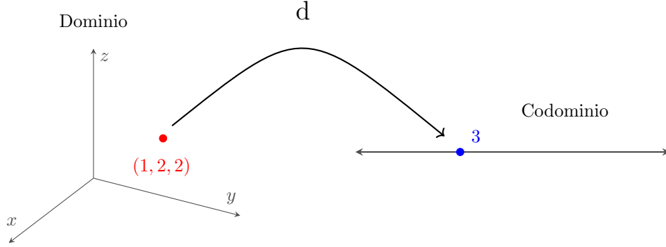
Figura 1.13: Visualización de (1, 2, 2) y d(1, 2, 2) = 3 .
