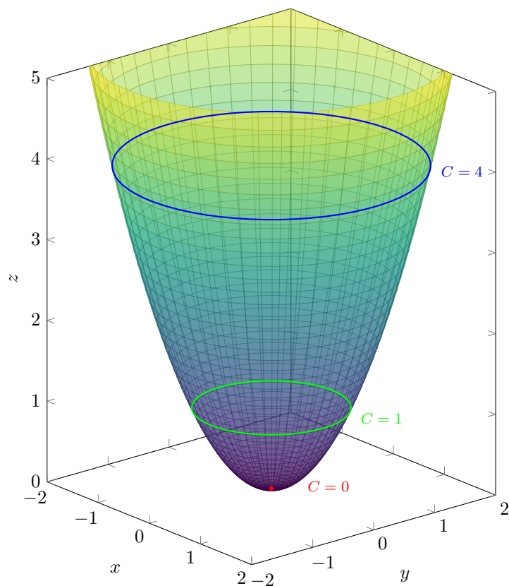
Figura 1.20: Gráfica de la función f .
