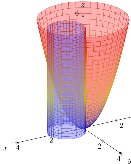
Figura 1.27: Representación de la región W . Ver en GeoGebra
