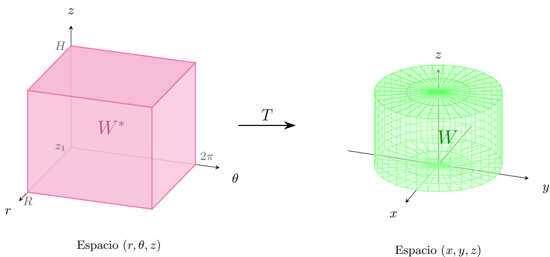
Figura 8.8: Visualización del sistema de coordenadas cilíndricas. El bloque W^* a la izquierda representa la región en el espacio (r, \theta, z) con sus límites típicos, mientras que el cilindro W a la derecha muestra cómo se transforma esa región en el espacio (x, y, z) mediante la transformación T . Ver en GeoGebra
