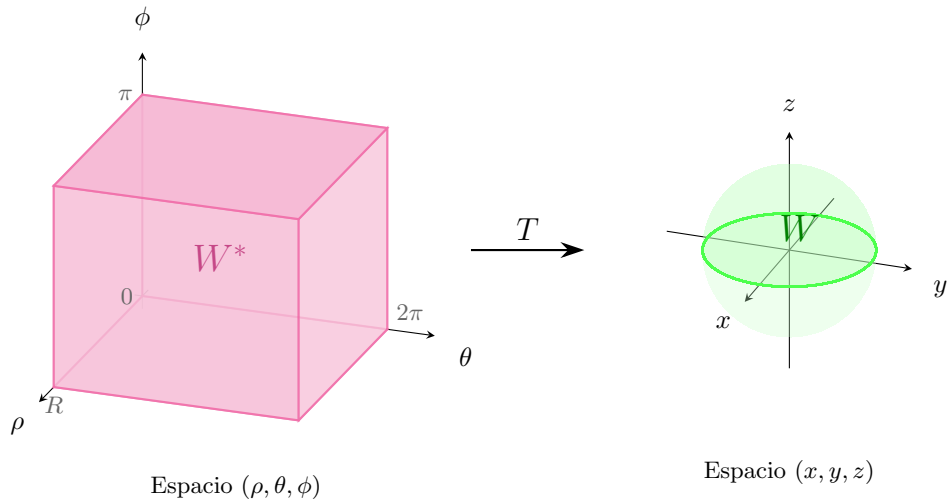
Figura 8.7: Visualización del sistema de coordenadas esféricas. El bloque W^* a la izquierda representa la región en el espacio (\rho, \theta, \phi) con sus límites típicos, mientras que la esfera W a la derecha muestra cómo se transforma esa región en el espacio (x, y, z) mediante la transformación T . Ver en GeoGebra
