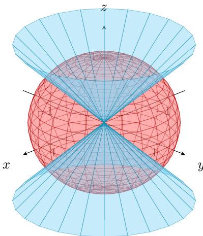
Figura 2.5: Representación de la región W . Ver en GeoGebra
