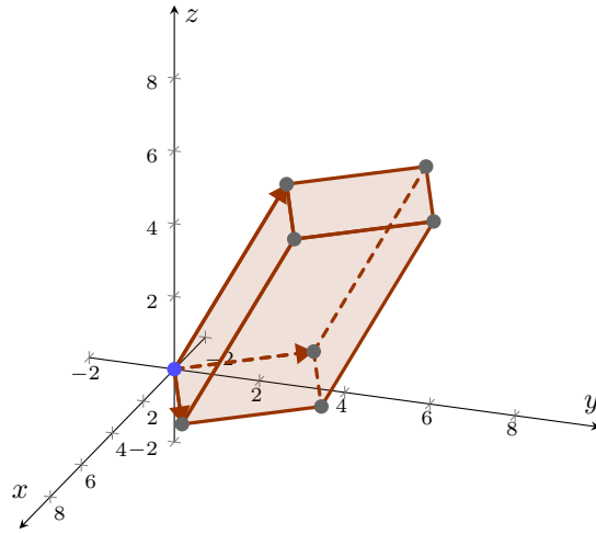
Figura 2.6: Representación de la región pedida. Ver en GeoGebra
