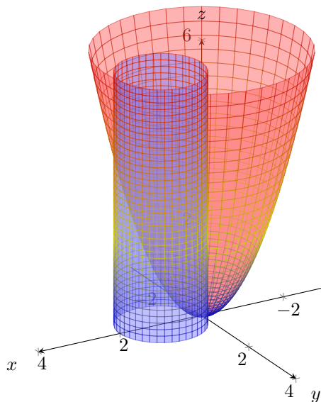
Figura 2.3: Representación de la región W . Ver en GeoGebra
