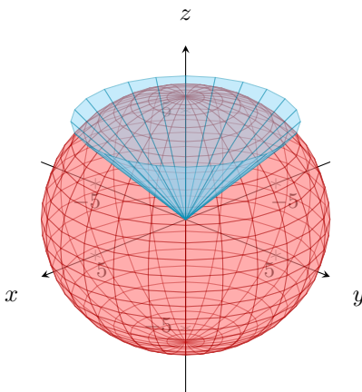
Figura 2.2: Representación de la región pedida. Ver en GeoGebra
