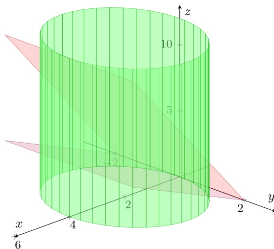
Figura 2.4: Representación de la región pedida. Ver en GeoGebra
