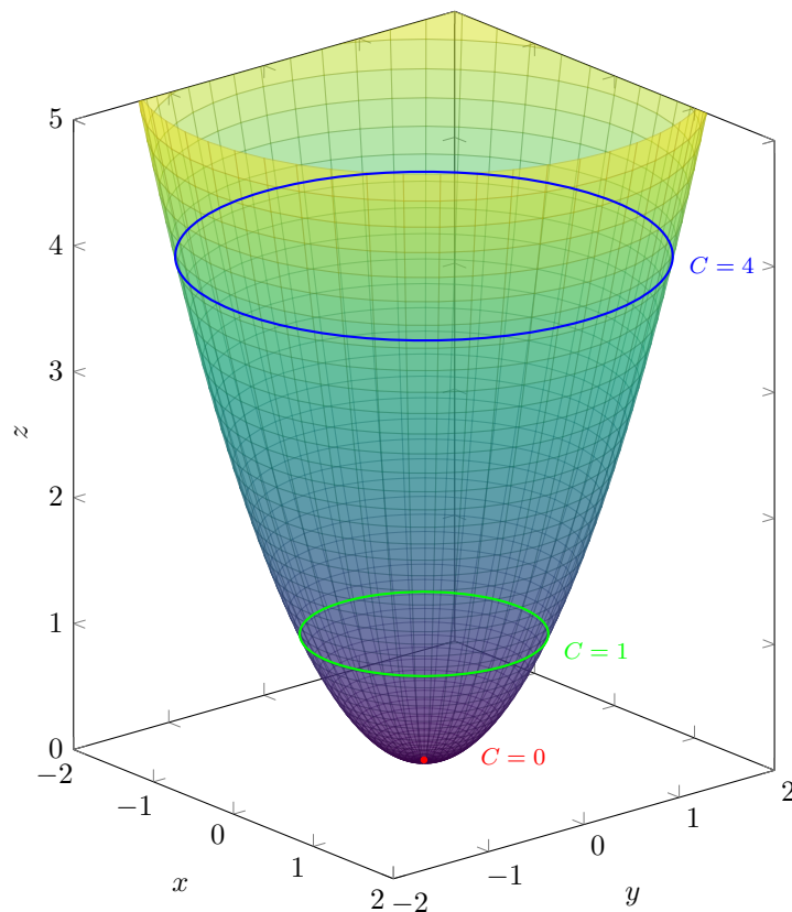
Figura 1.20: Gráfica de la función f .
