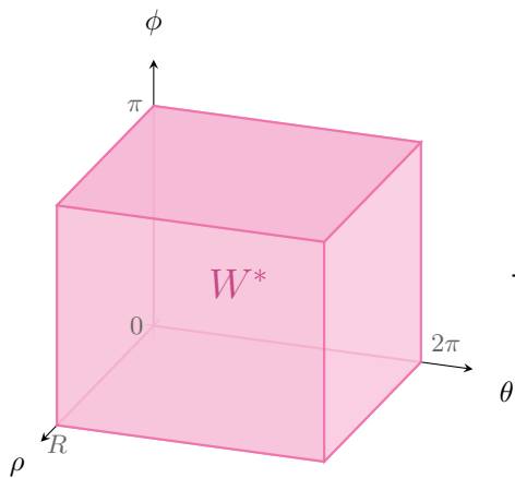
Espacio (\rho, \theta, \phi)
