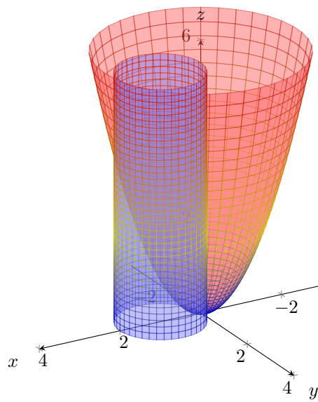
Figura 8.8: Representación de la región W . Ver en GeoGebra
