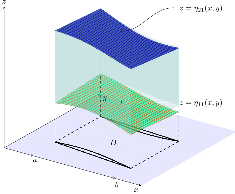
Figura 8.2: Conjunto elemental de Tipo I.
