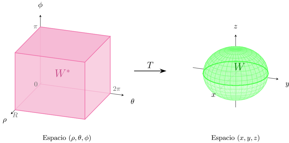
Figura 8.6: Visualización del sistema de coordenadas esféricas. El bloque W^* a la izquierda representa la región en el espacio (\rho, \theta, \phi) con sus límites típicos, mientras que la esfera W a la derecha muestra cómo se transforma esa región en el espacio (x, y, z) mediante la transformación T . Ver en GeoGebra
