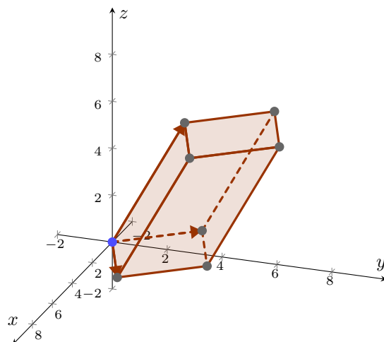
Figura 8.12: Representación de la región pedida. Ver en GeoGebra
