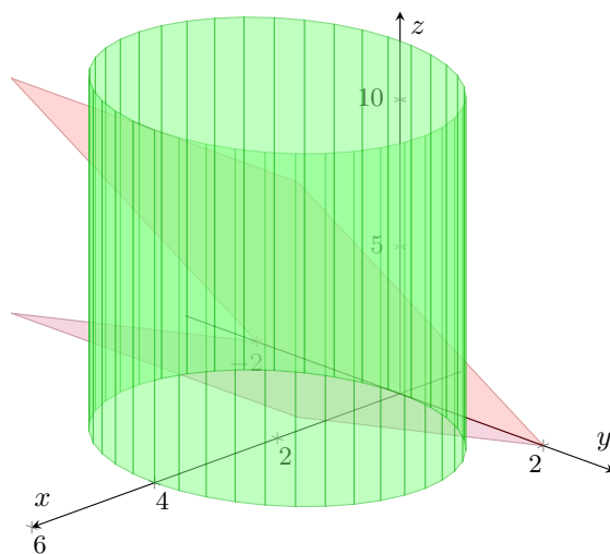
Figura 8.10: Representación de la región pedida. Ver en GeoGebra
