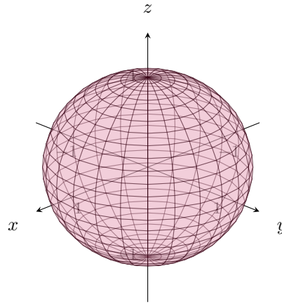
Figura 8.5: Representación de la región W .
