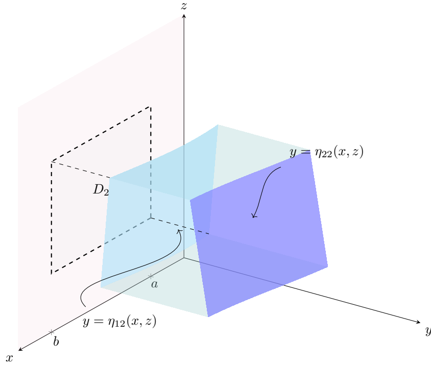
Figura 8.3: Conjunto elemental de Tipo 2.
