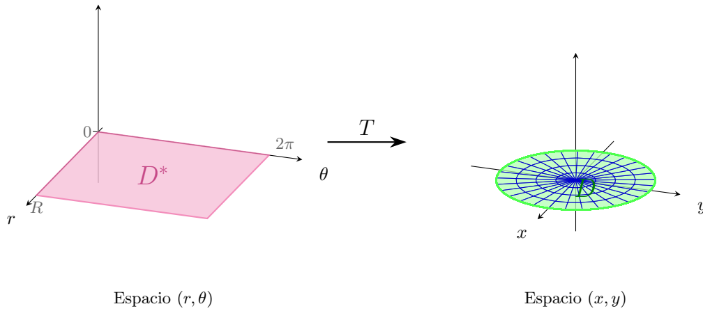
Figura 8.1: Visualización del sistema de coordenadas polares. El bloque D^* a la izquierda representa la región en el espacio (r, \theta) con sus límites típicos, mientras que el disco D a la derecha muestra cómo se transforma esa región en el espacio (x, y) mediante la transformación T .
