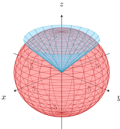
Figura 8.8: Representación de la región pedida. Ver en GeoGebra
