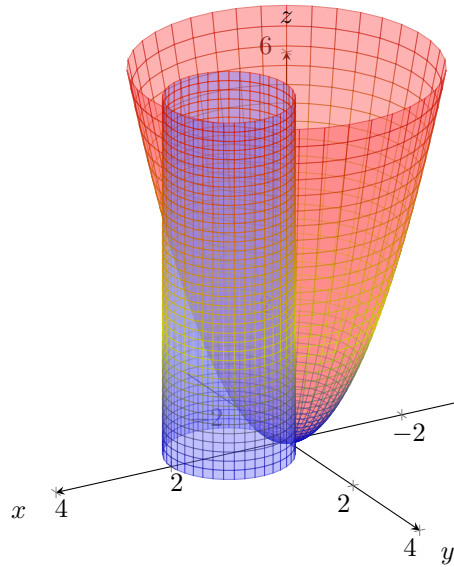
Figura 8.9: Representación de la región W . Ver en GeoGebra
