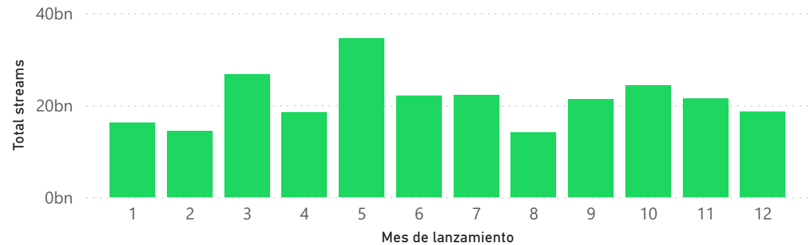
Total streams por mes de lanzamiento
