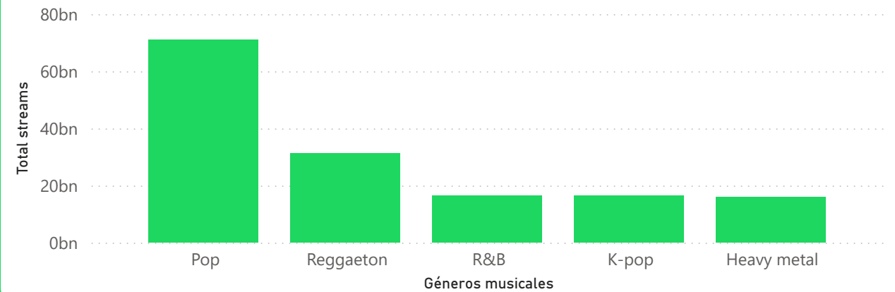
Total streams por género
