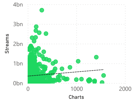
Charts por streams
