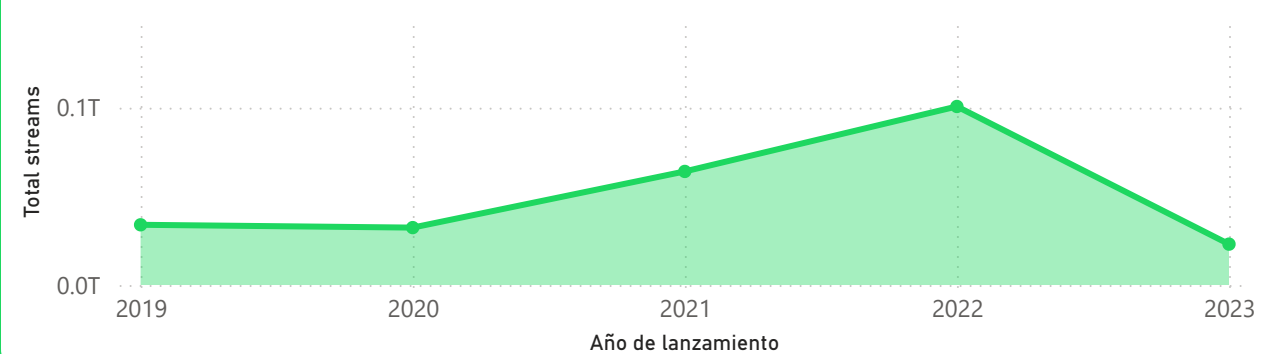
Total streams por año de lanzamiento
