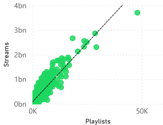
Playlists por streams
