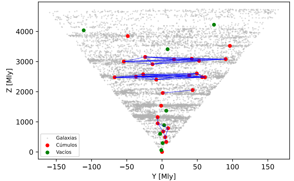
Red Cósmica Completa - Proyección YZ
