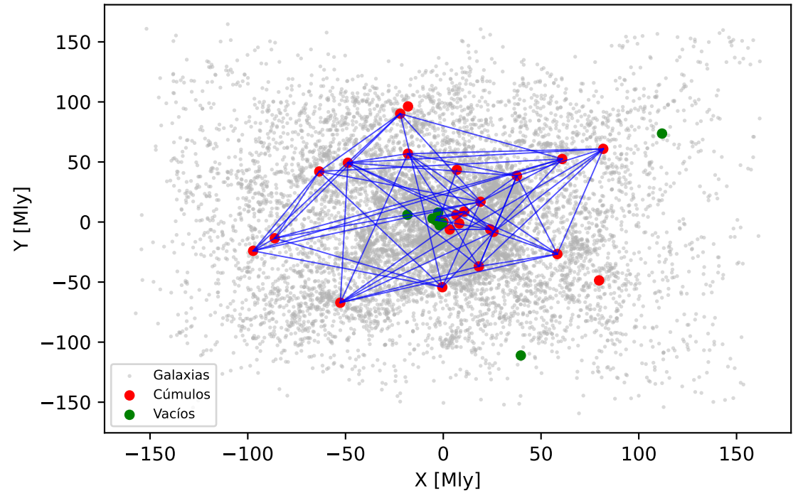
Red Cósmica Completa - Proyección XY
