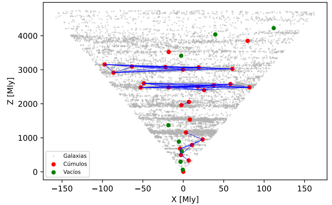
Red Cósmica Completa - Proyección XZ
