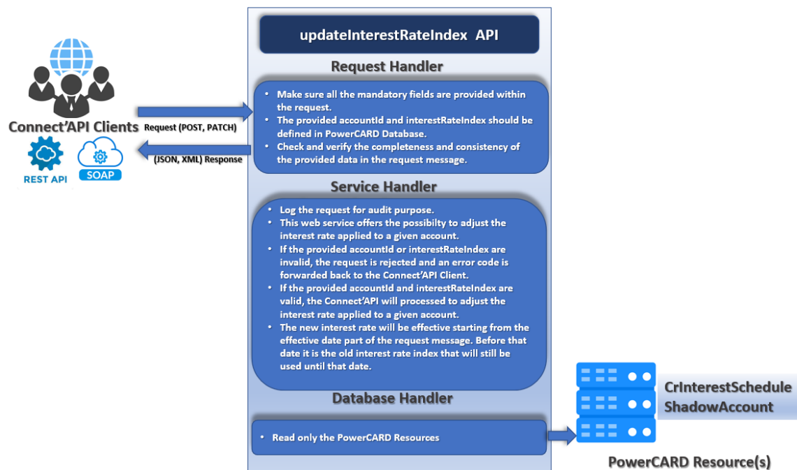
Figure 66: updateInterestRateIndex process
