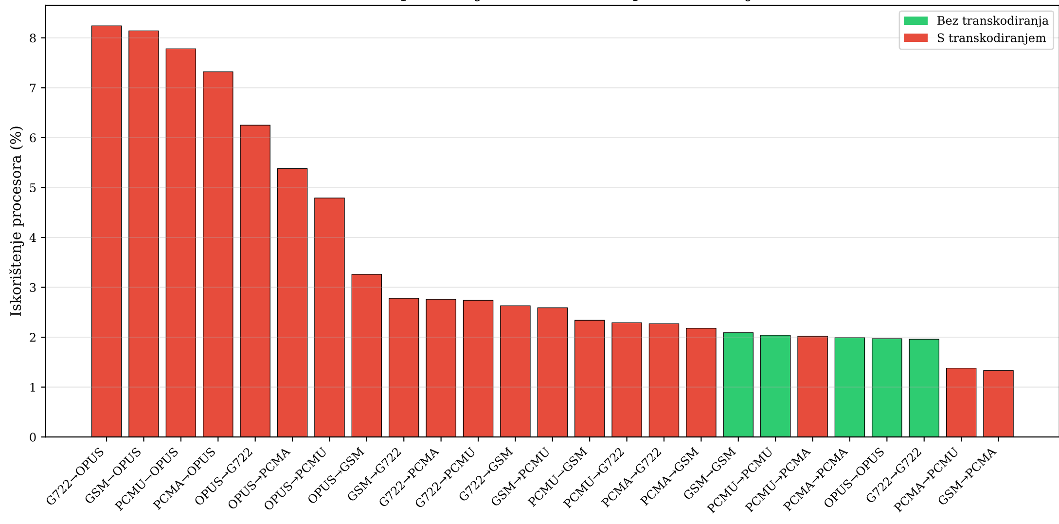
Procesorsko opterećenje FreeSWITCH-a po kombinaciji kodeka
