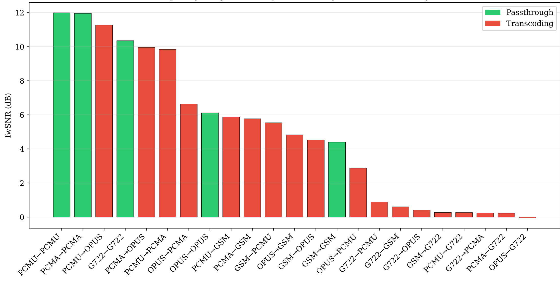
Frequency-Weighted SNR po kombinaciji kodeka (više = bolje)
