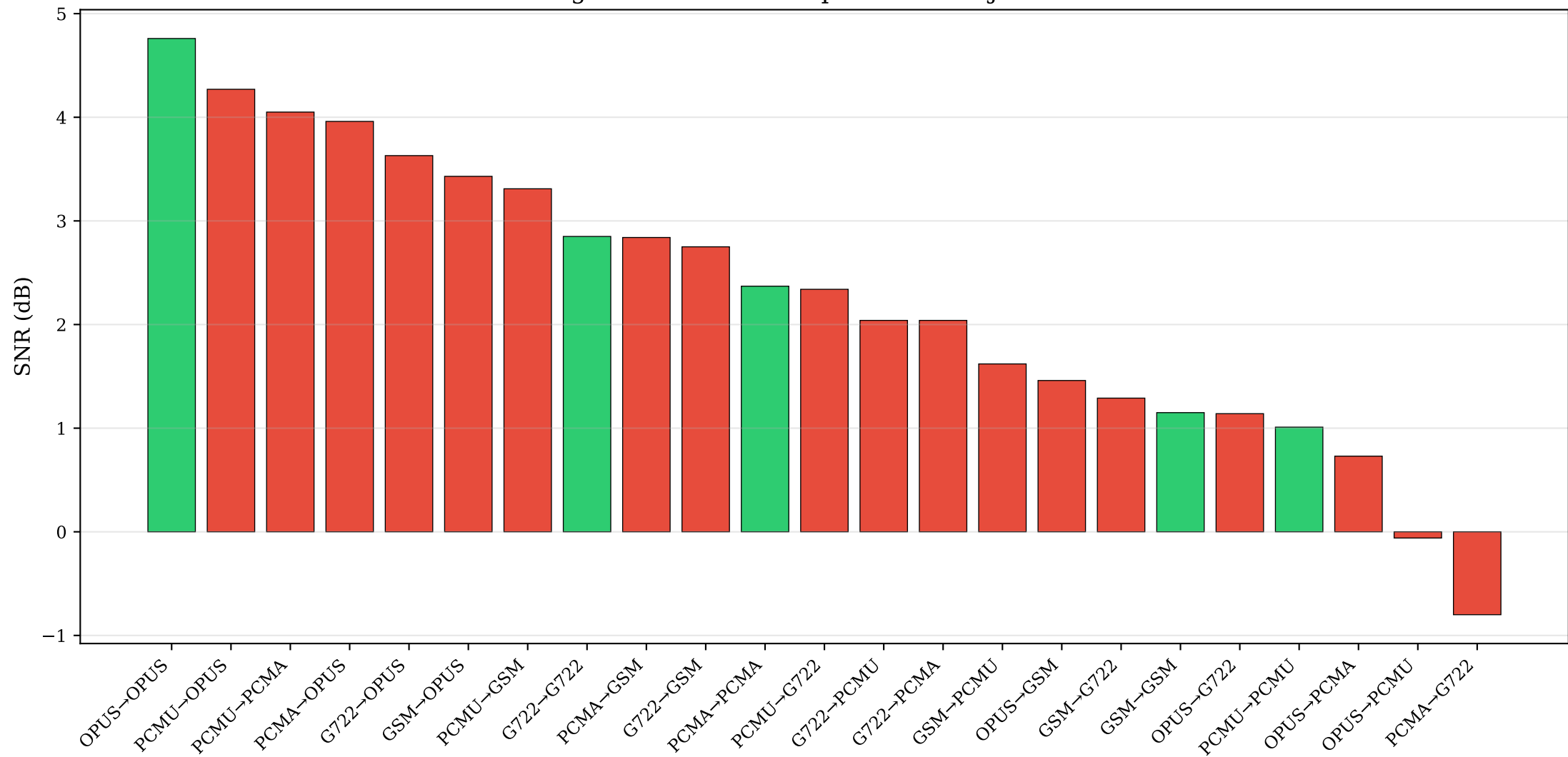
Signal-to-Noise Ratio po kombinaciji kodeka
