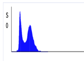
S0Histo
