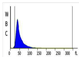
WBCHisto
