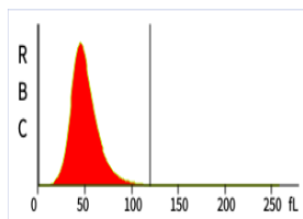
RBCHisto
