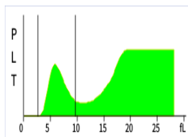
PLTHisto
