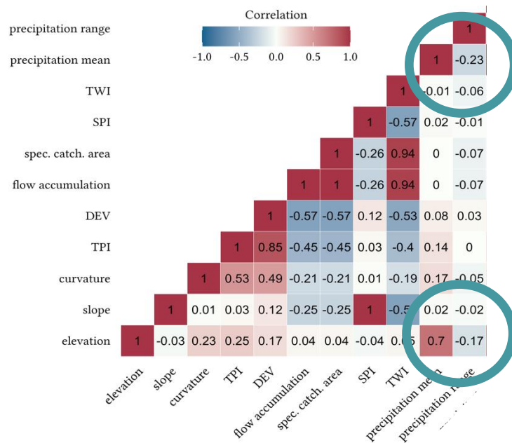
After FST
