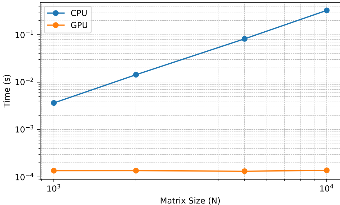
SpMV: CPU vs GPU Time
