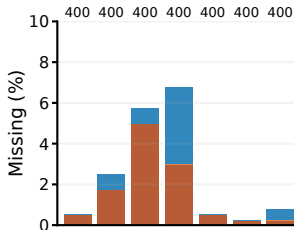
Gemma-4-12B-IT
