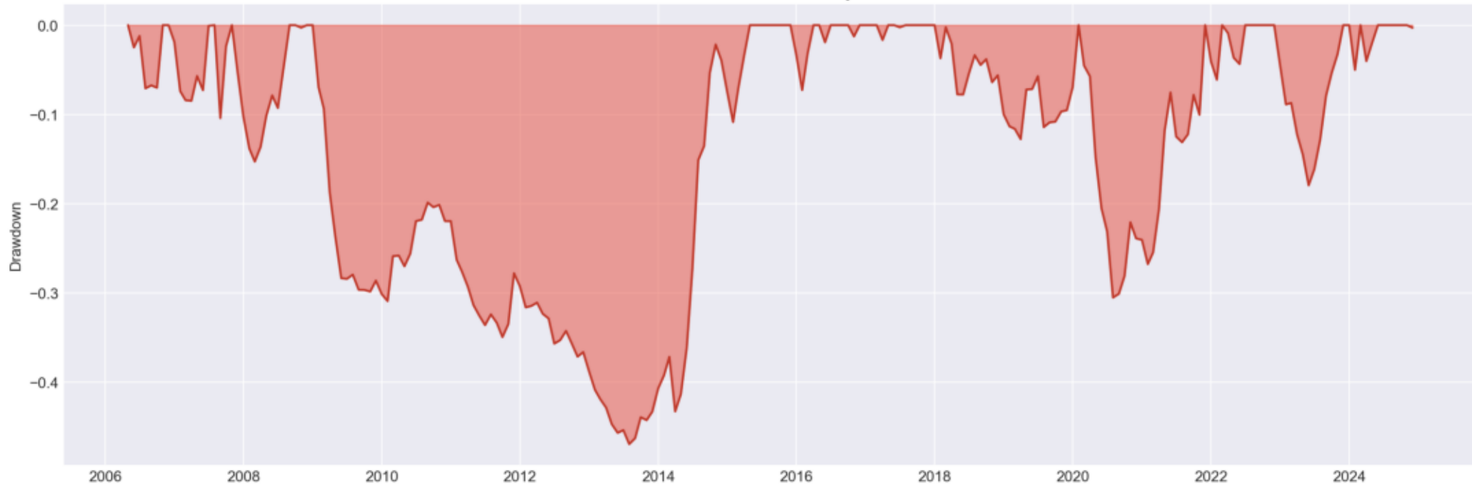
Drawdown — mlp
