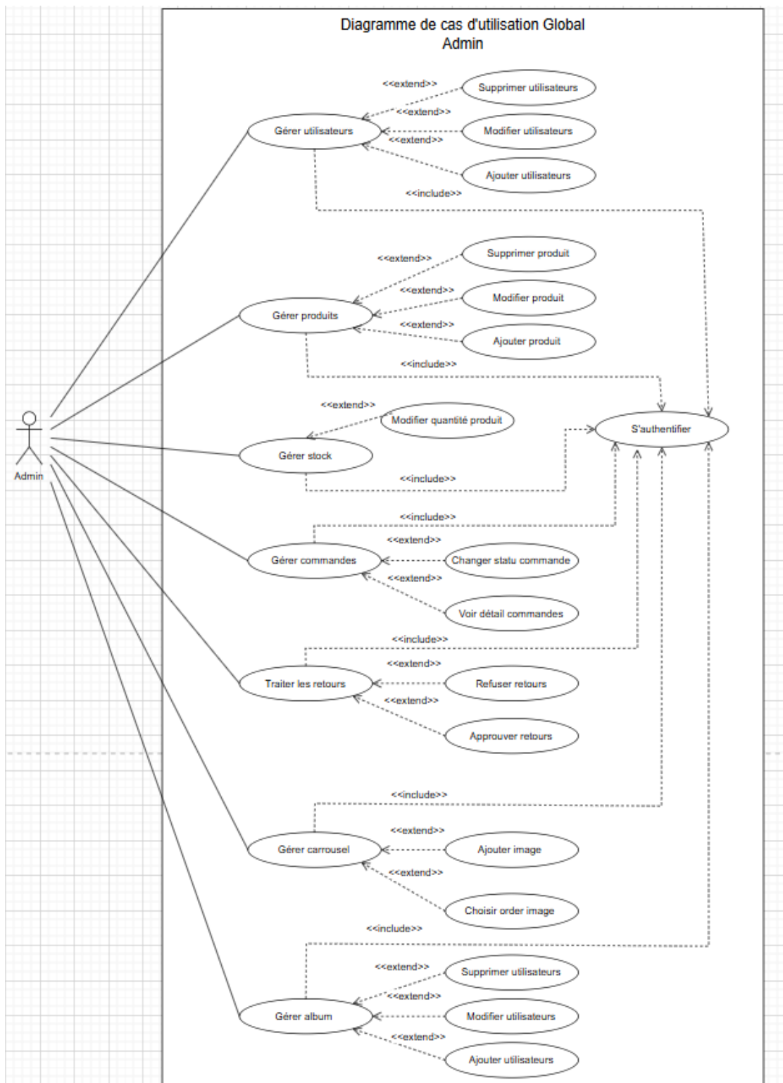
Figure 8 : Diagramme de cas d'utilisateur partie admin
