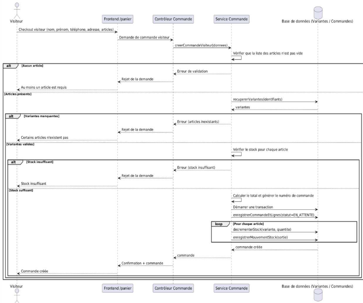
Figure 16 : Diagramme de Séquence Passage de commande (visiteur)
