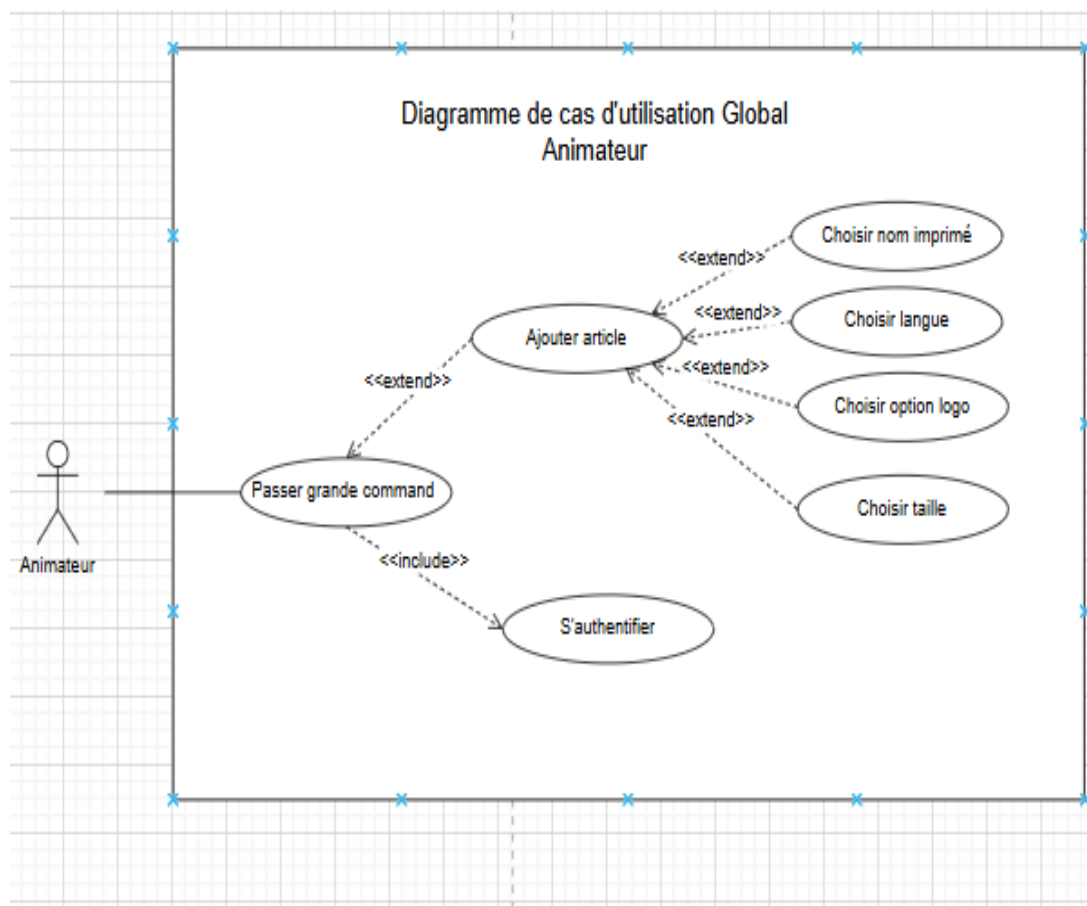
Figure 9 : Diagramme de cas d'utilisateur partie animateur
