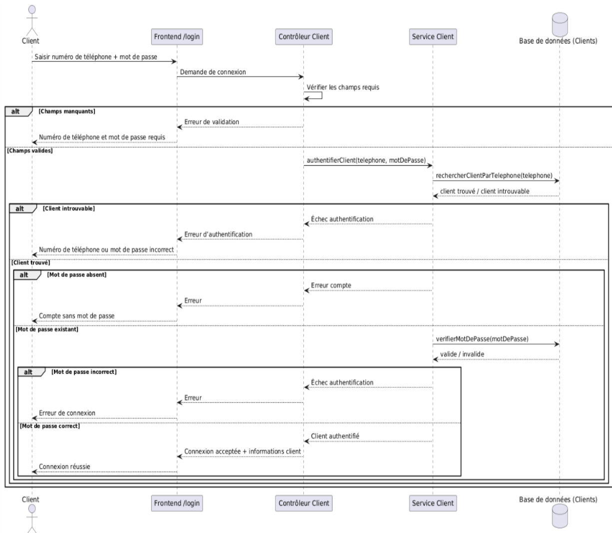
Figure 14 : Diagramme de Séquence Login
