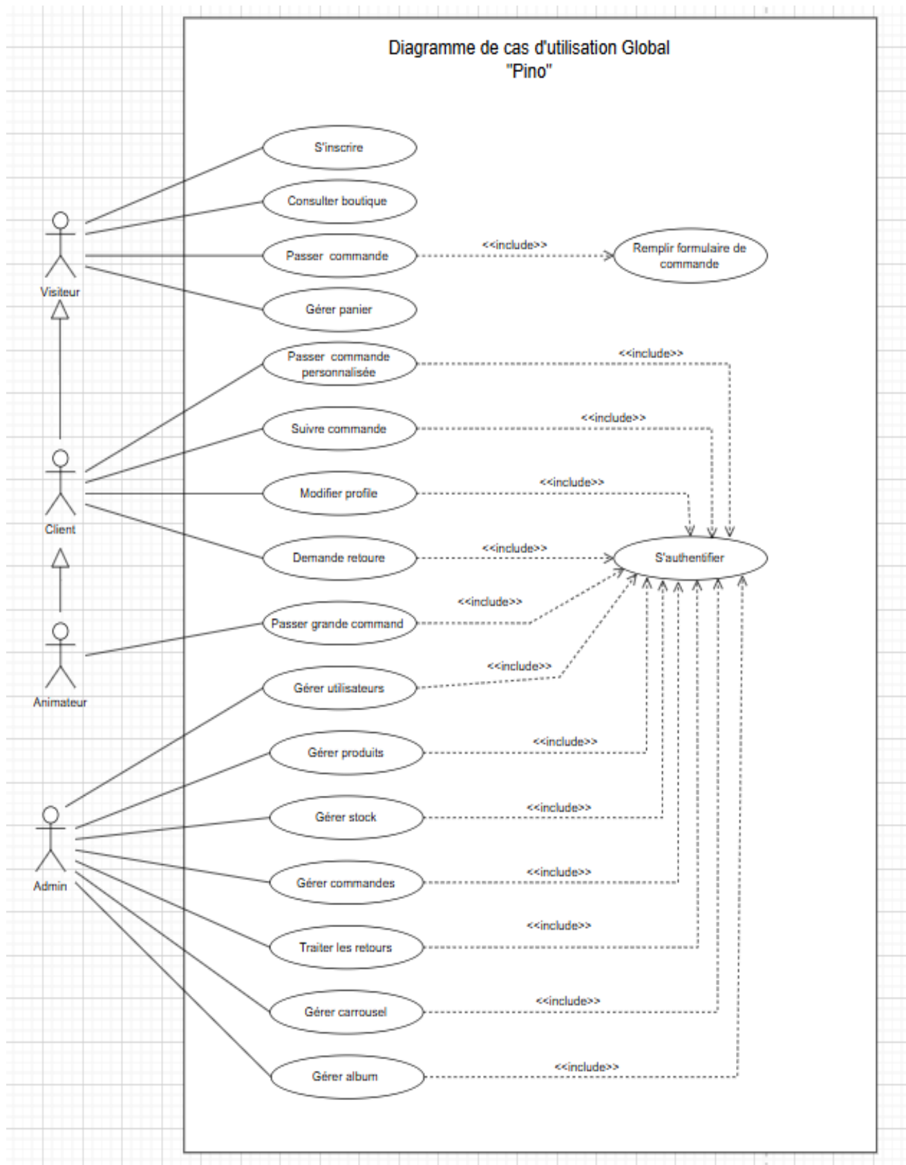
Figure 5 : Diagramme de cas d'utilisateur
