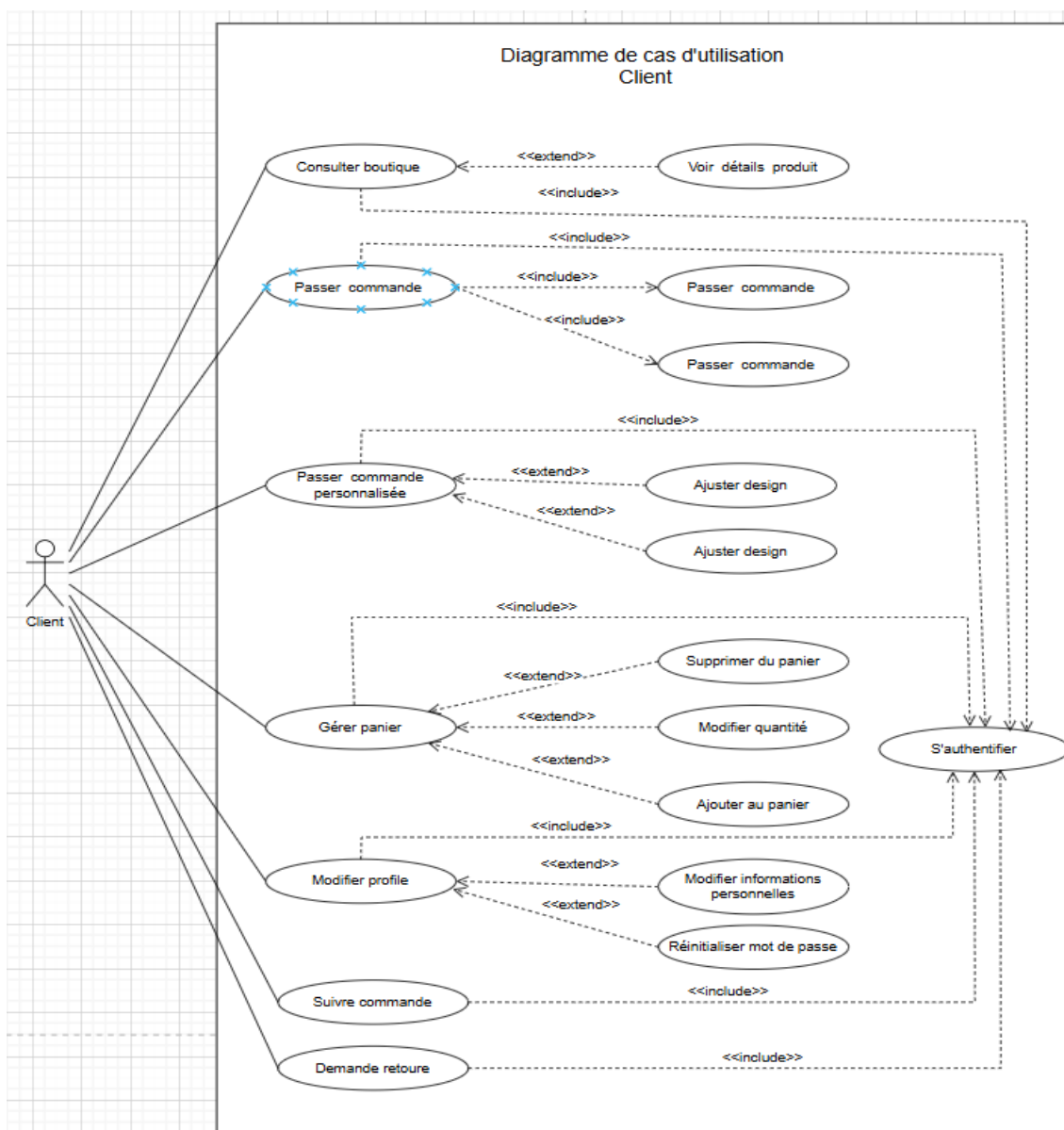
Figure 6 : Diagramme de cas d'utilisateur partie client
