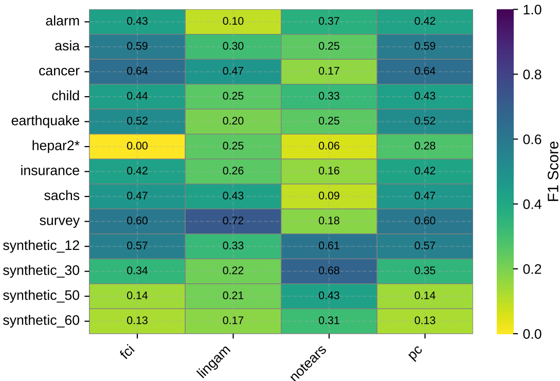
F1 Score: Dataset vs Algorithm
