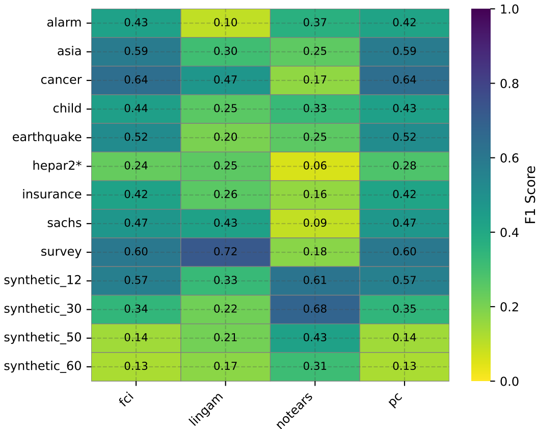
F1 Score: Dataset vs Algorithm
