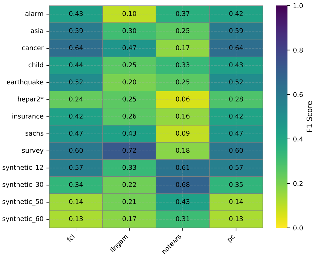
F1 Score: Dataset vs Algorithm
