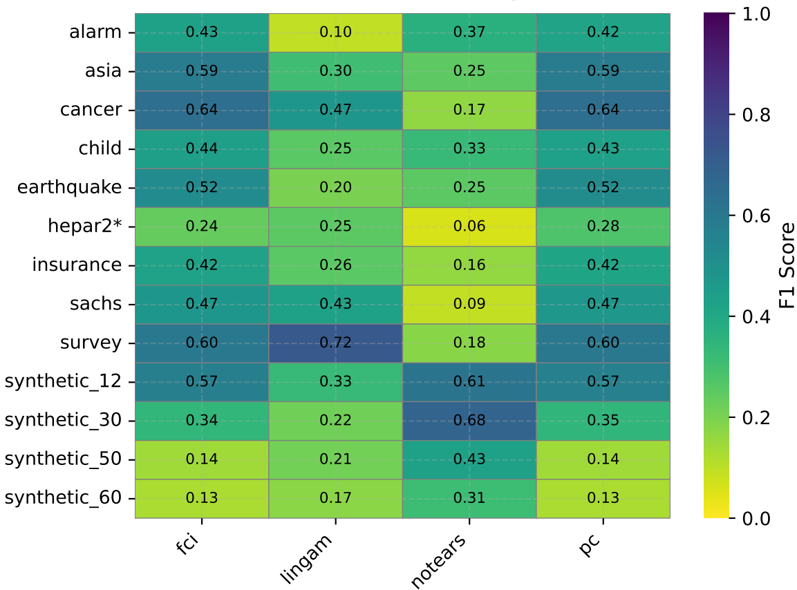
F1 Score: Dataset vs Algorithm
