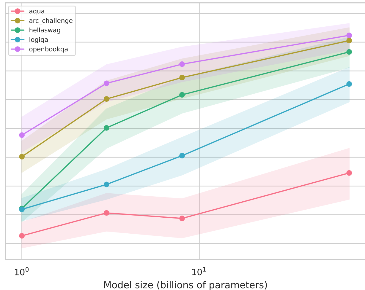
Llama family
