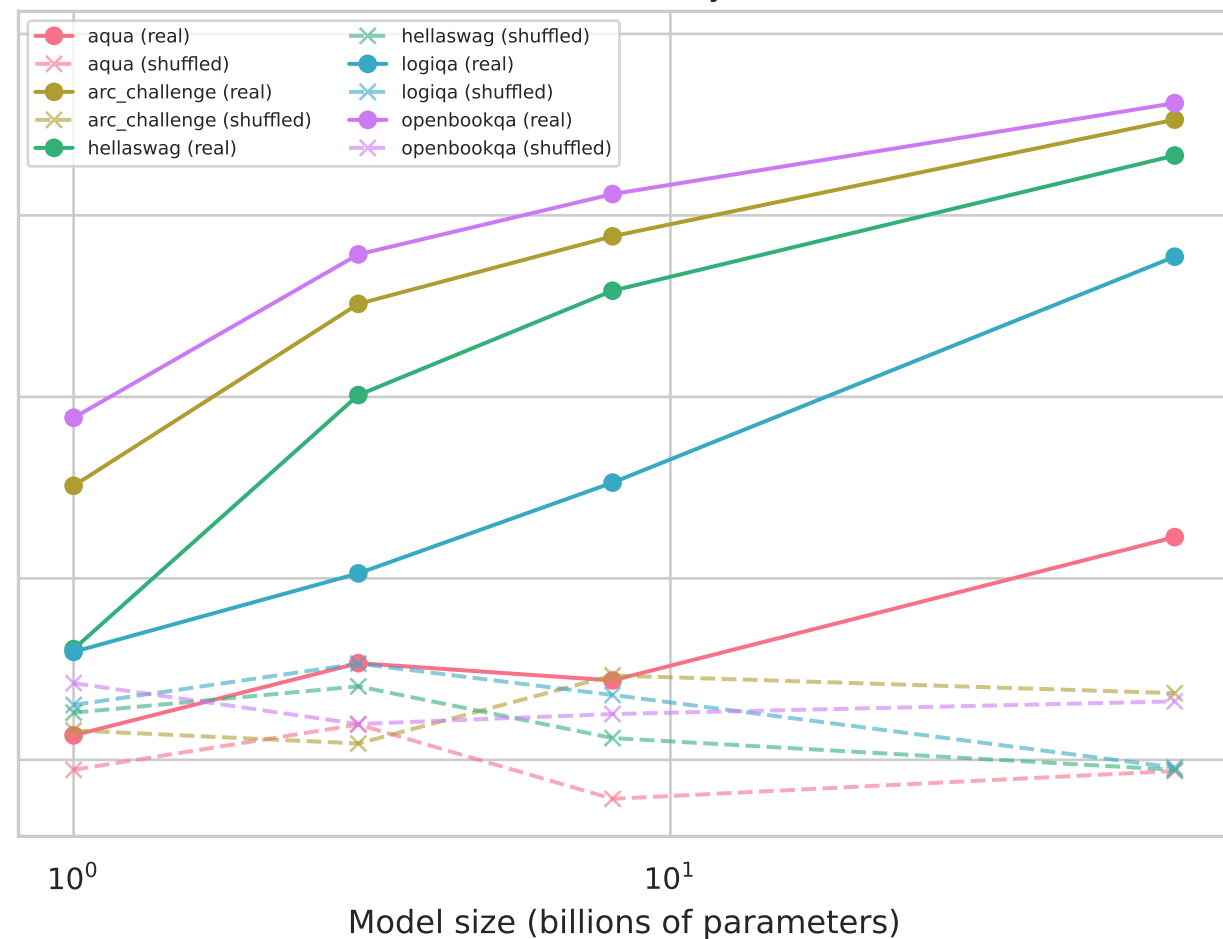
Llama family
