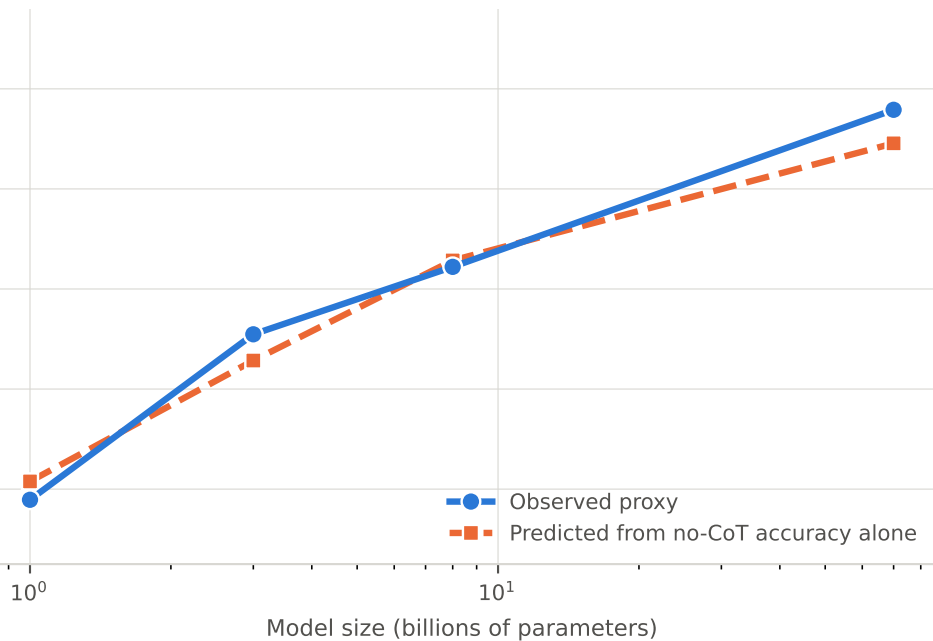
Llama-3-Instruct
